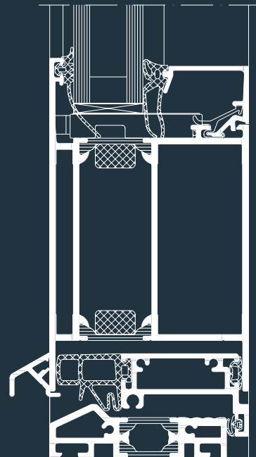
Schüco Tür ADS 75 HD.HI, Fußpunkt, Maßstab 1:2 Schüco Door ADS 75 HD.HI, Sill, Scale 1:2
